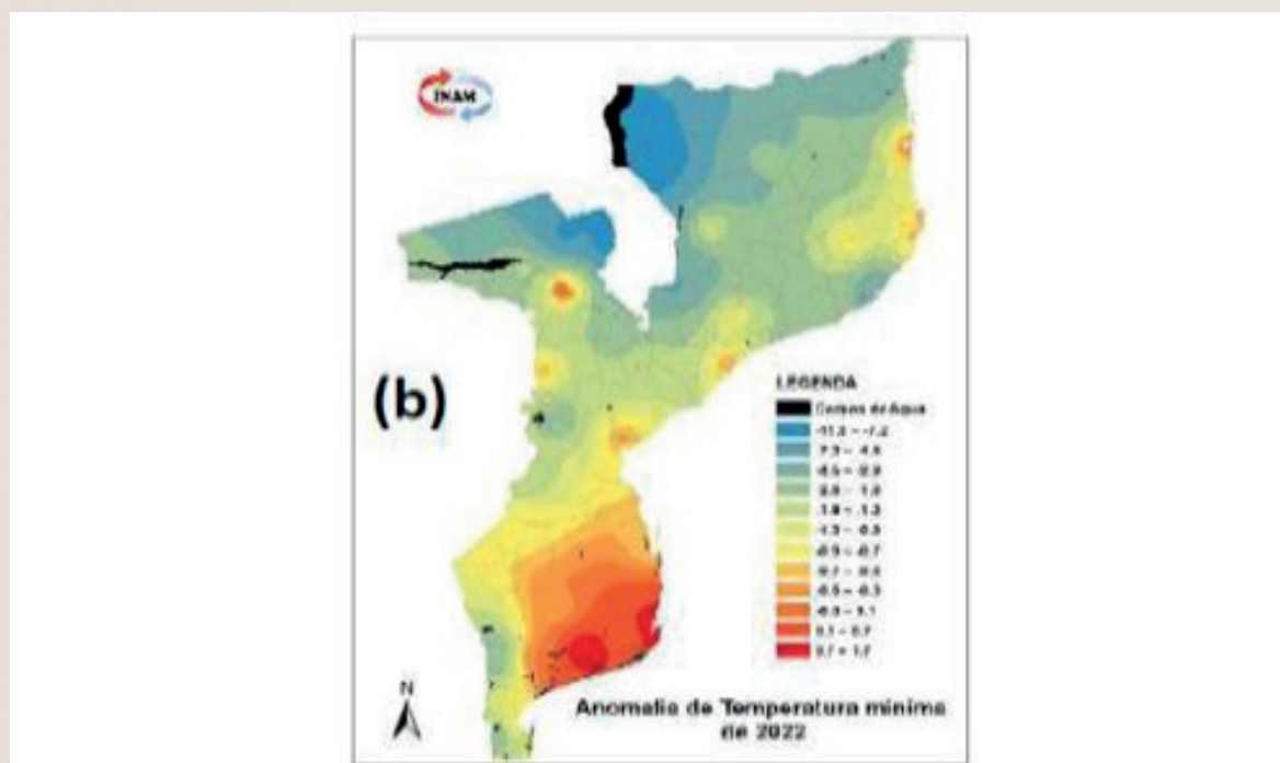
Figura 3. Anomalia da temperatura mínima
