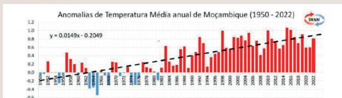
Figura 1. Anomalia da temperatura média em Moçambique. Fonte: (INAM, 2023).
