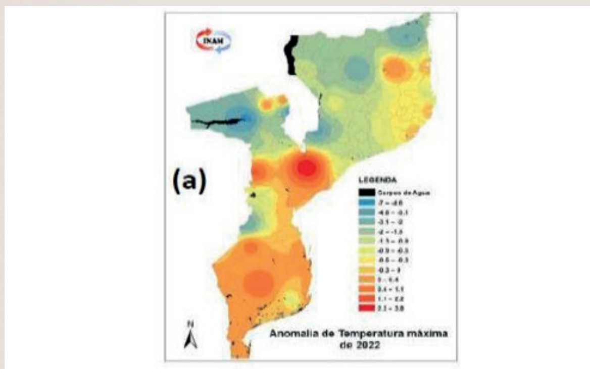
Figura 2. Anomalia da temperatura máxima
